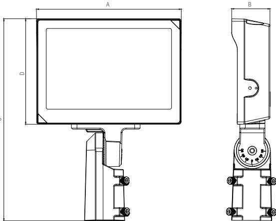
Slipfitter
