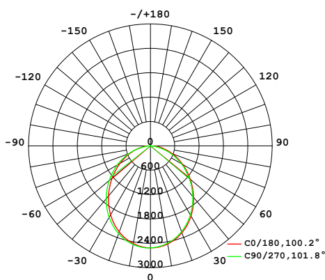
SP-12E 4000K-48W
