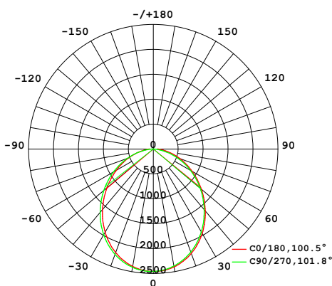
SP-12E 3000K-48W
