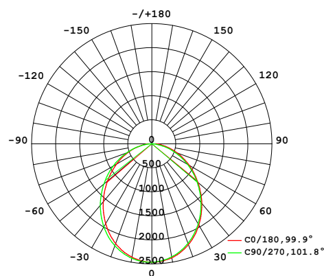
SP-12E 5000K-48W
