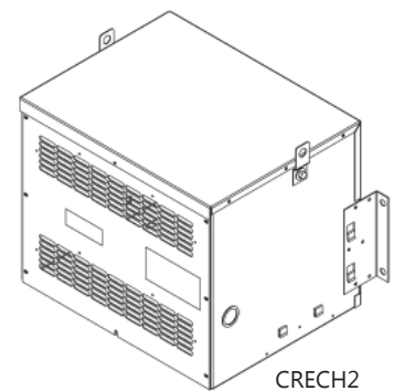
CH2
