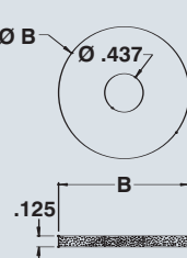
NEOPRENE GASKET
