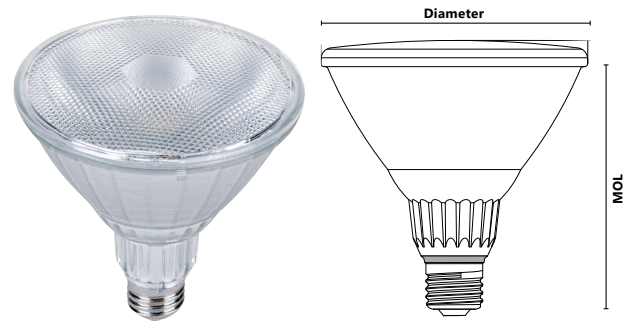
MOL: 5" (127 mm) Dia.: 4 23/32" (120 mm)
