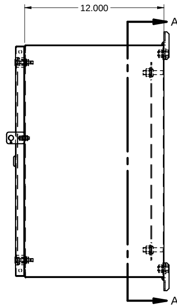
SIDE / CÔTÉ
