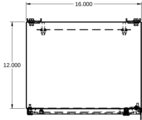
TOP / DESSUS
