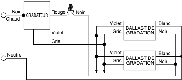
Figure 2 – câblage 3 voies
