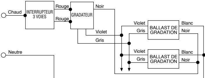
Figure 2 – câblage 3 voies
