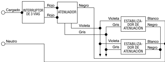
Figura 2 – Cableado de 3 vías
