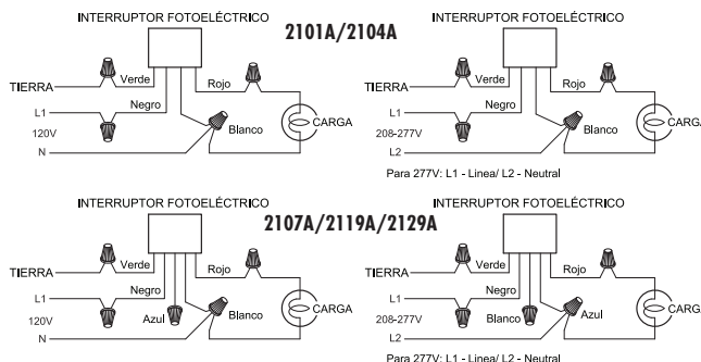
DIAGRAMA DE CABLEADO
