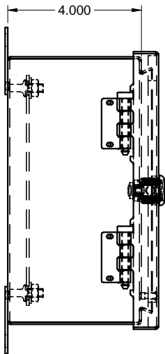
SIDE / CÔTÉ
