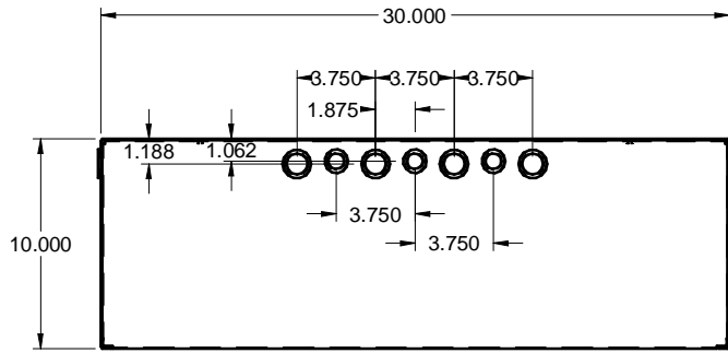
TOP / DESSUS
