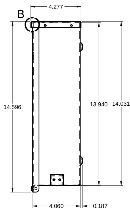
SIDE / CÔTÉ
