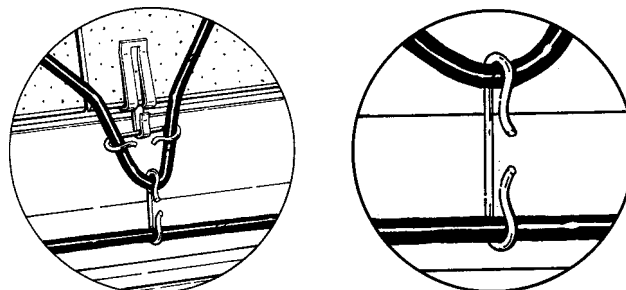
Figure 19. Fixer les pinces dans les gouttières
