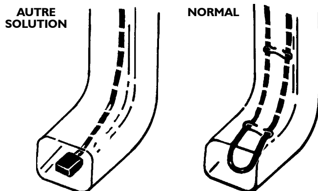
Figure 22. Câble dans les descentes pluviales de « bout du parcours »
