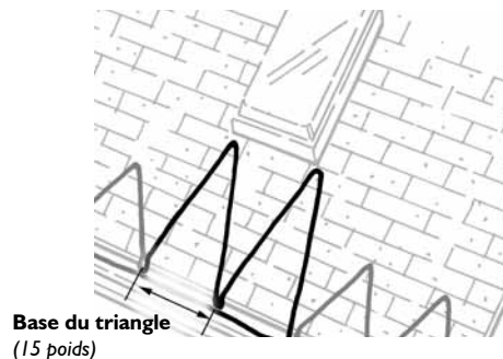
Figure 5. Parcours du triangle près d'un puits de lumière
