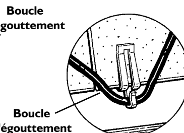
Figure 14. Fixer les pinces aux bandeaux au niveau de la bordure du toit sans gouttières
