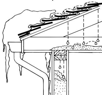
Figure A-2. La formation d'un banc de glace et ses conséquences
