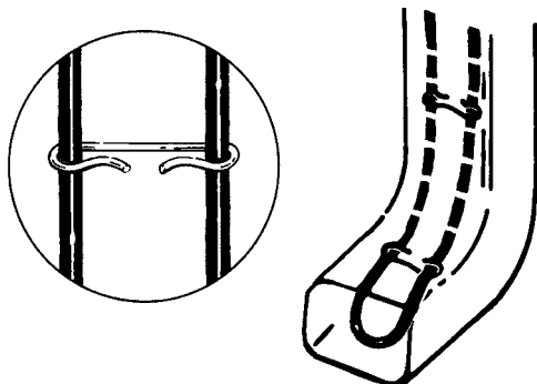
Figure 21. Double parcours de câble dans les descentes pluviales le « long du parcours »
