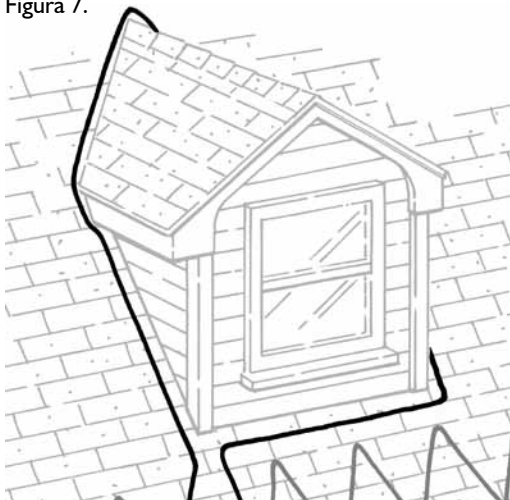
Figura 7. Diseño del recorrido del cable alrededor de las buhardillas Modelo ADKS guía del usuario
