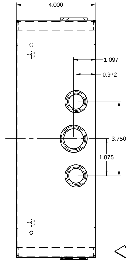
SIDE / CÔTÉ
