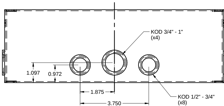
BOTTOM / DESSOUS
