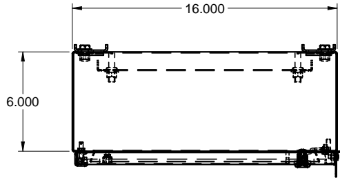
TOP / DESSUS
