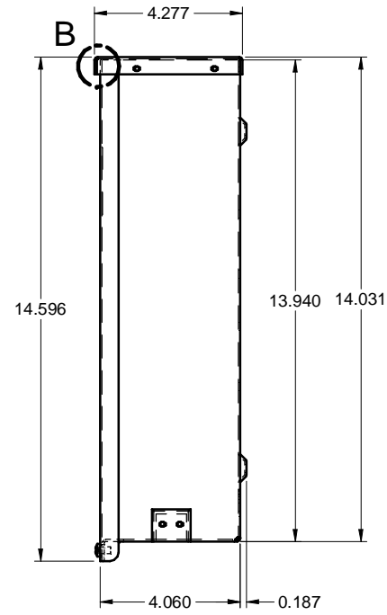
SIDE / CÔTÉ
