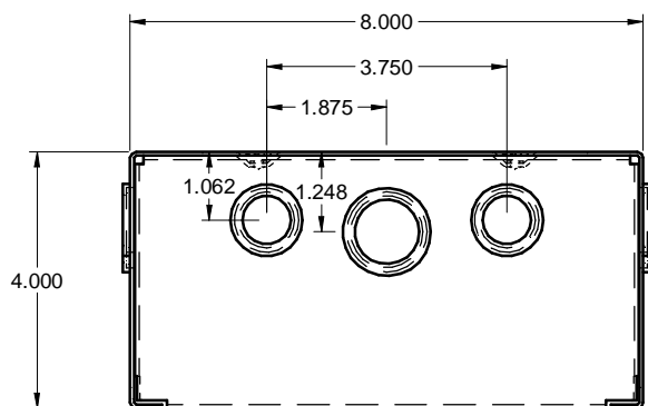
TOP / DESSUS
