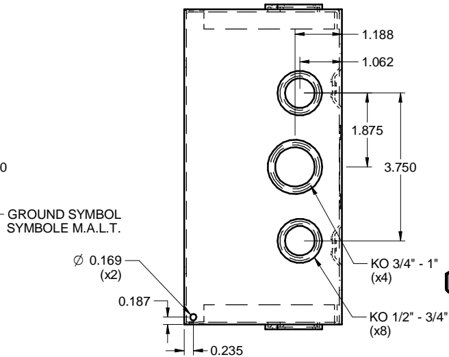
SIDE / CÔTÉ
