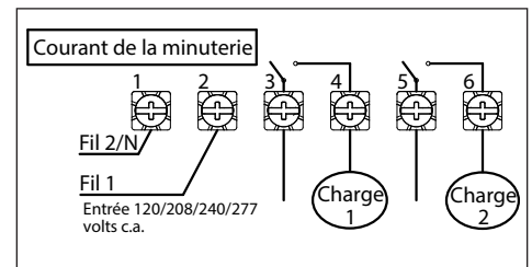
La minuterie ET8215 est configurée pour deux impulsions unipolaires unidirectionnelles (SPST) avec le cavalier réglé sur IND
