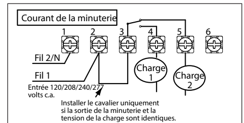
La minuterie ET8115 est configurée pour une commutation de charge unipolaire bidirectionnelle (SPDT)
