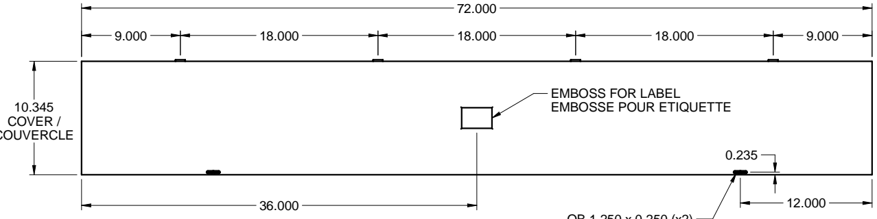
TOP / DESSUS
