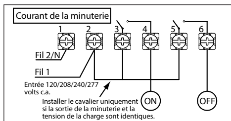
La minuterie ET1125 est configurée pour une impulsion unipolaire unidirectionnelle (SPST) avec le cavalier réglé sur PUL
