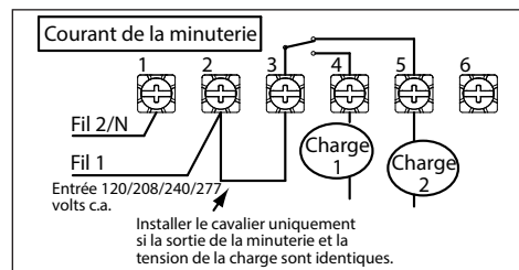
La minuterie ET1115 est configurée pour une commutation de charge unipolaire bidirectionnelle (SPDT)
