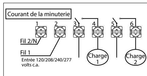
La minuterie ET1125 est configurée pour deux impulsions unipolaires unidirectionnelles (SPST) avec le cavalier réglé sur IND
