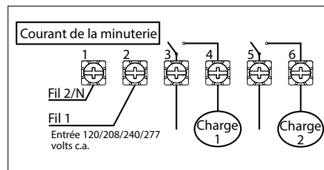
La minuterie ET1125 est configurée pour une communication bipolaire unidirectionnelle (DPST) avec le cavalier réglé sur SIM
