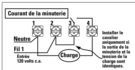
ET1105 configuré pour unipolaire unidirectionnel (SPST), charge 120 V c.a.
