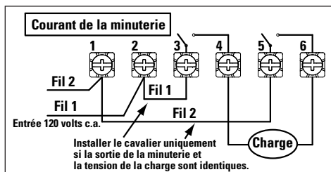
La minuterie ET1125 est configurée pour une communication de charge 240 V c.a. bipolaire unidirectionnelle (DPST) avec le cavalier réglé sur SIM
