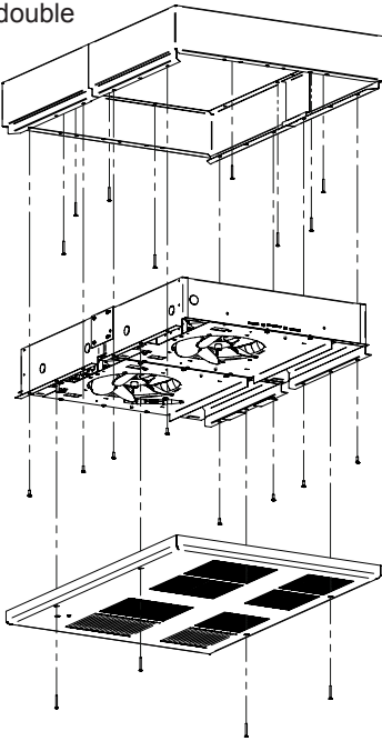
Montage en surface Unité double
