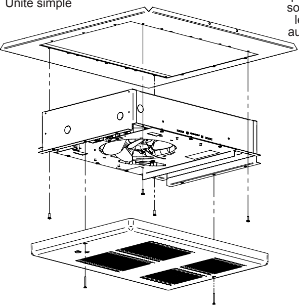
Cadre d’installation pour plafond suspendu Unité simple
