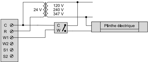
Schéma de branchement pour une plinthe électrique
