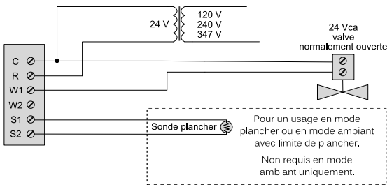
Schéma de branchement pour une valve d'eau chaude
