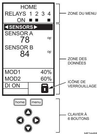
Fig. 24. Affichage à Cristaux Liquid (ACL) - Écran d'accueil et clavier.
