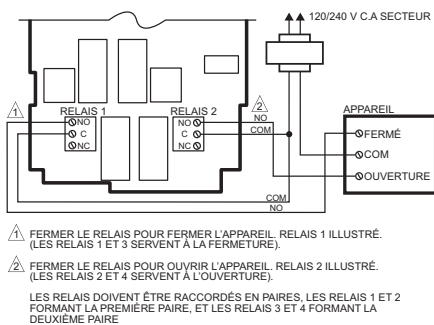
Fig. 14. Raccordement d'une sortie flottante (paire formée par le relais 1 et le relais 2 illustrée).
