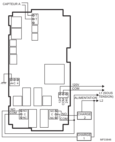
Fig. 10. Raccordement électrique d'un régulateur à deux étages - 120 (entrée de 120 V c.a. et charge de 120 V c.a. illustrées).
