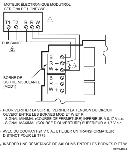
Fig. 19. Raccordement d'un moteur Modutrol série 90.
