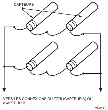
Fig. 3. Raccordement de capteurs en séries parallèles.
