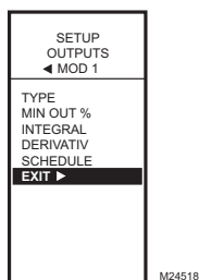
Fig. 55. Configuration - Sorties - Sortie modulante - Quitter.
