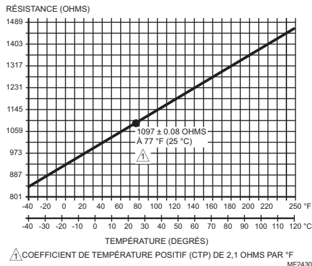
Fig. 23. Résistance du capteur par rapport à la température.
