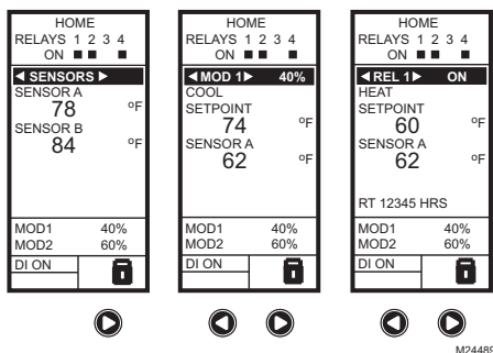
Fig. 25. Affichage cristaux liquides - Écran d'accueil affichant les capteurs, les sorties modulantes et les relais actifs.
