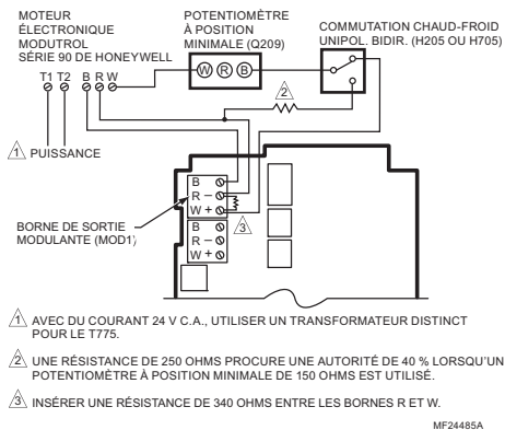
Fig. 20. Raccordement d'un relais de commutation et d'un potentiomètre à position minimale utilisés avec des moteurs Modutrol série 90.
