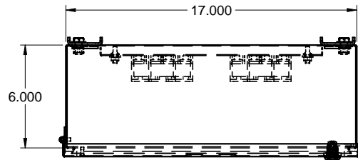
TOP / DESSUS
