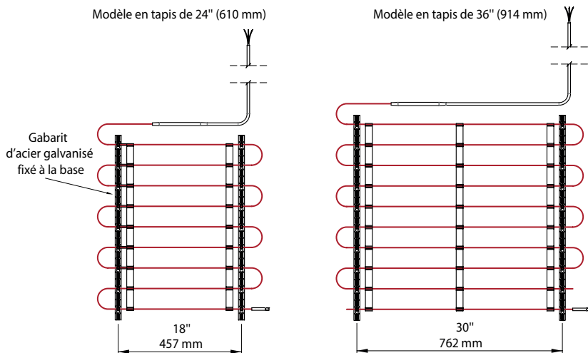
Figure 3 : Positionnement du gabarit
