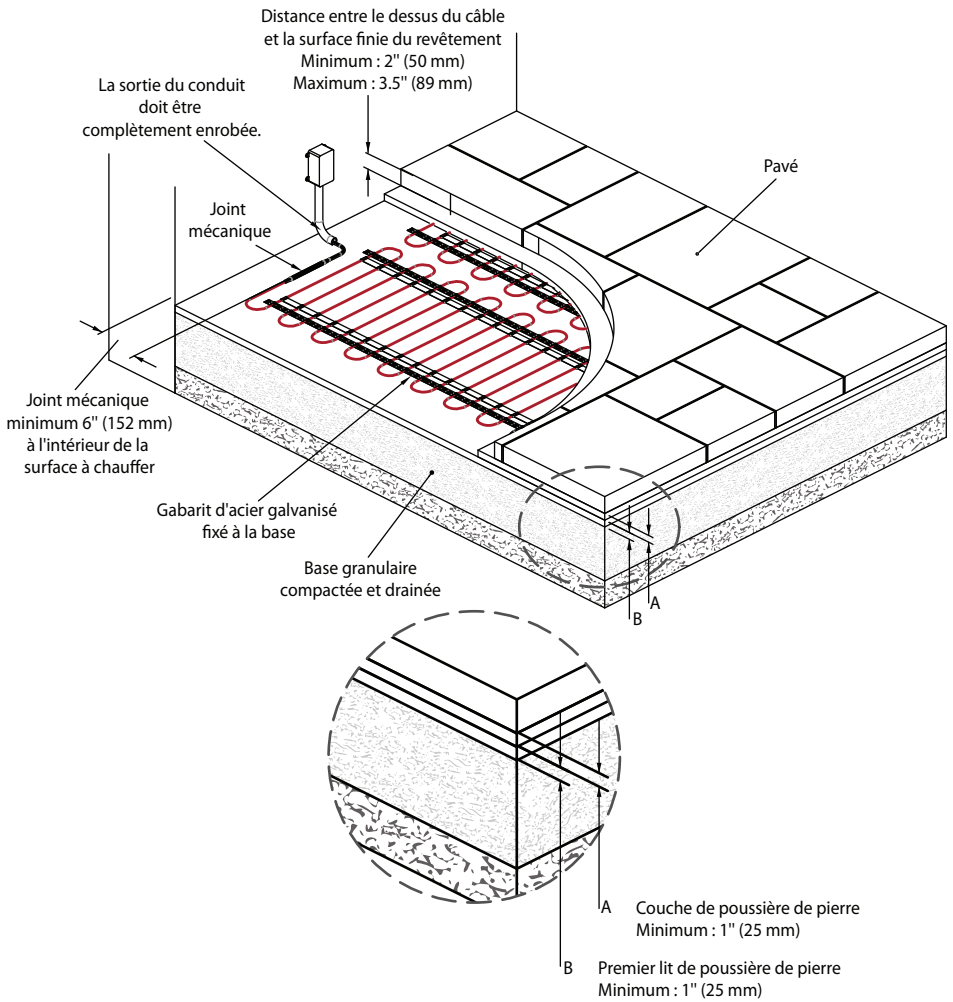
Figure 11 : Revêtement de pavé de brique, de béton ou de pierre naturelle
