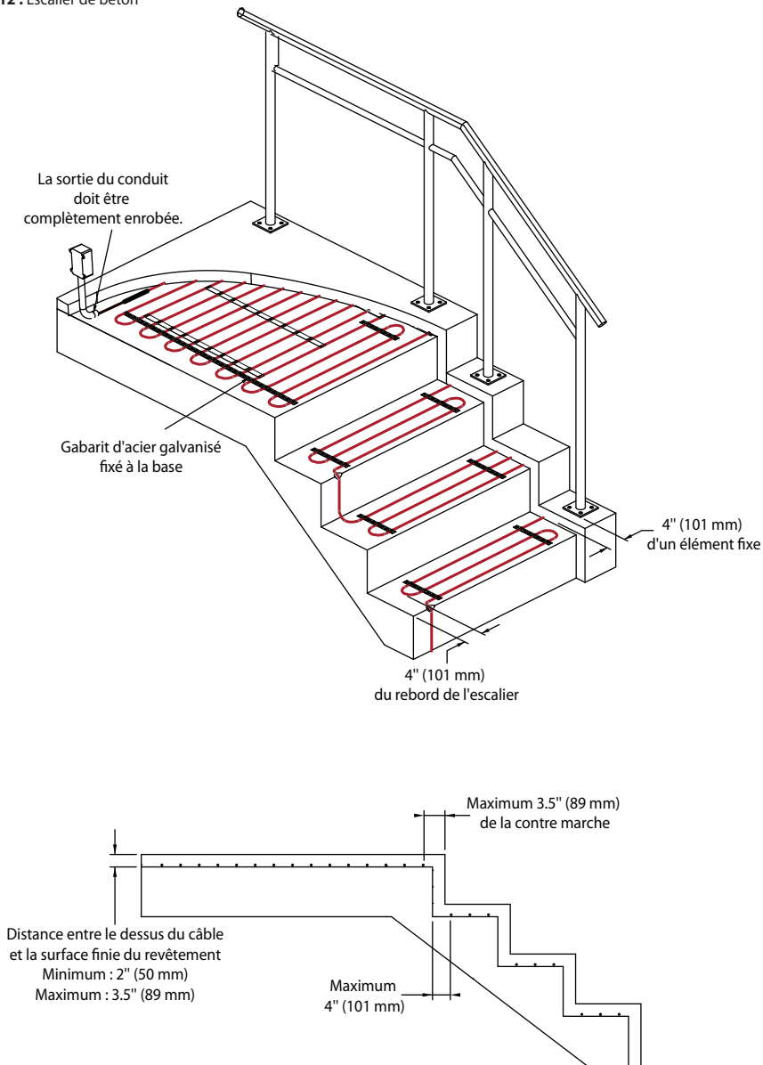
Figure 12 : Escalier de béton
