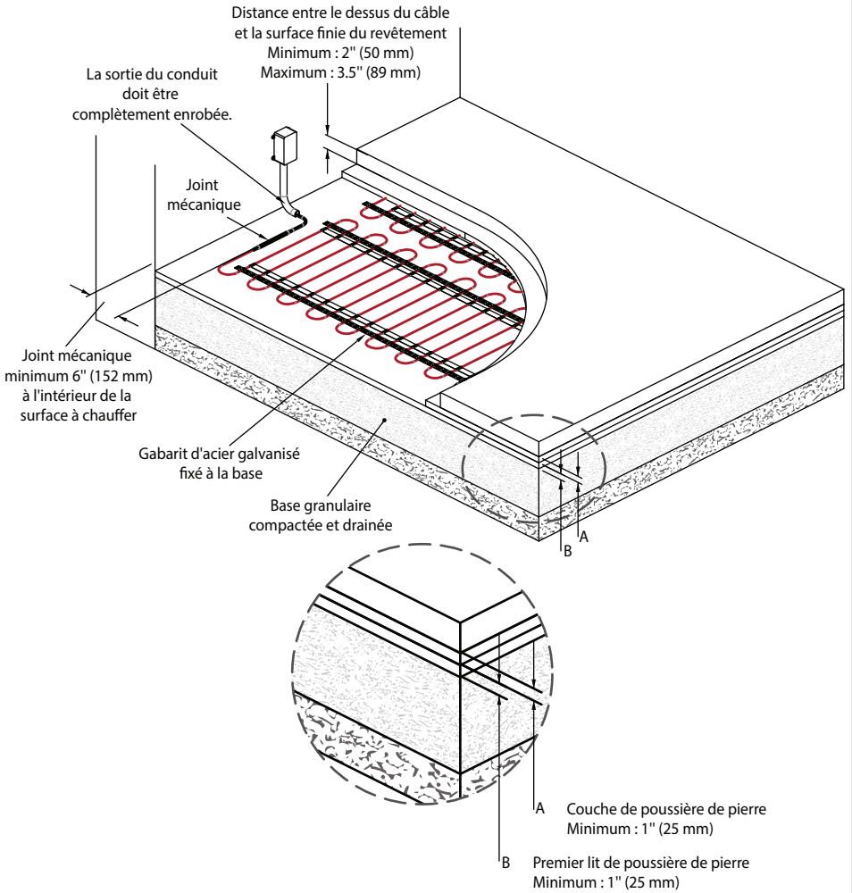
Figure 10 : Revêtement d'asphalte (une coulée, câbles chauffants enrobés de poussière de pierre)
