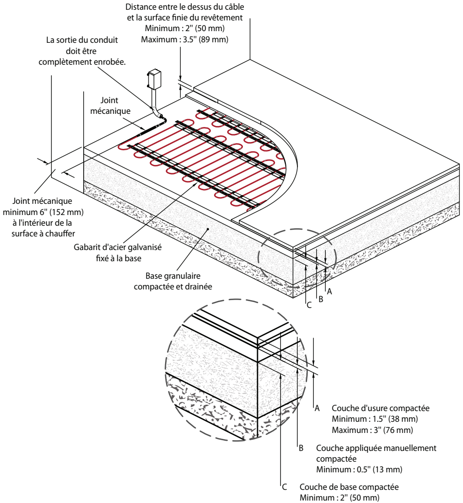
Figure 9 : Revêtement d'asphalte (deux coulées)
