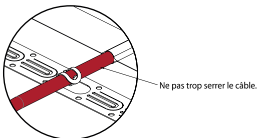
Figure 4 : Méthode de fixation du câble au gabarit
