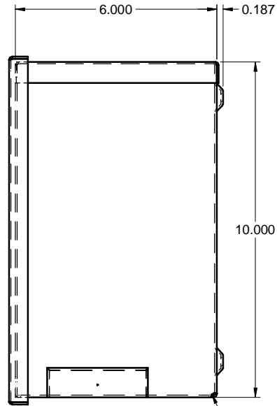
SIDE / CÔTÉ
