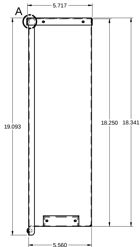
SIDE / CÔTÉ
