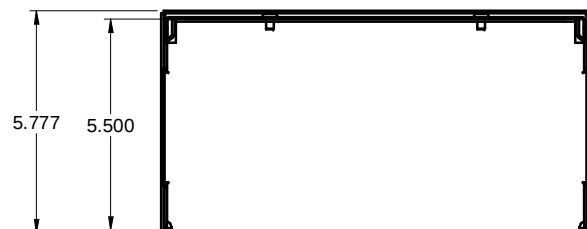
BOTTOM / DESSOUS
