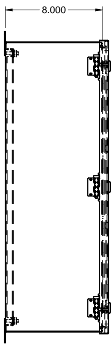
SIDE / CÔTÉ
