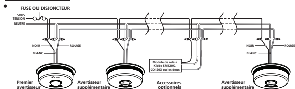
Schéma de câblage d'interconnexion
