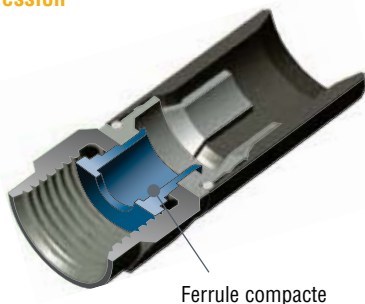
Ferrule compacte
