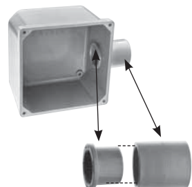
Adaptateur pour boîte de jonction Manchon standard en PVC
