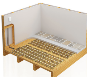
OWC-M : Installation sous une chape de béton de 1.5 à 4 po
