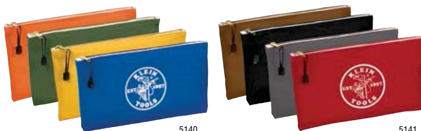
5140
