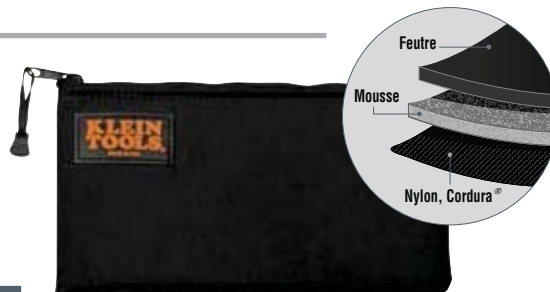
5139PAD
