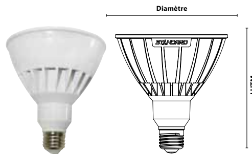
LHTM : 5 po (127 mm) Dia. : 4 23/32 po (120 mm)
