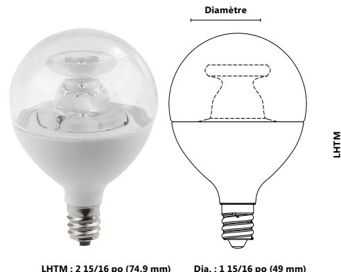
LHTM : 2 15/16 po (74.9 mm) Dia. : 1 15/16 po (49 mm)
