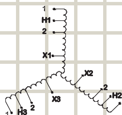
Configuration optionnelle avec prises \pm 1 \times 5 %
