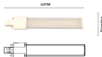
LHTM : 7 3/32 po. (180.5 mm) Dia. : 1 5/16 po. (33 mm)
