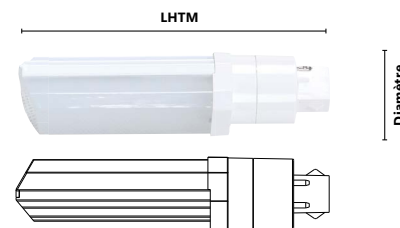
LHTM : 5 3/16 po (132 mm) Dia. : 1 1/8 po (41 mm)
