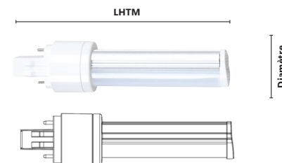
LHTM : 5 13/16 po. (147.5 mm) Dia. : 1 13/32 po. (35.5 mm)
