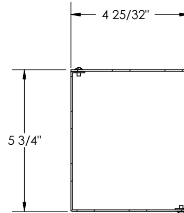
SECTION A-A SCALE 1 : 4
