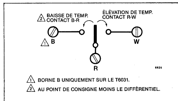
FIG. 5 — BORNES DE RACCORDEMENT DES RÉGULATEURS DE TEMPÉRATURE T4031 ET T6031.
