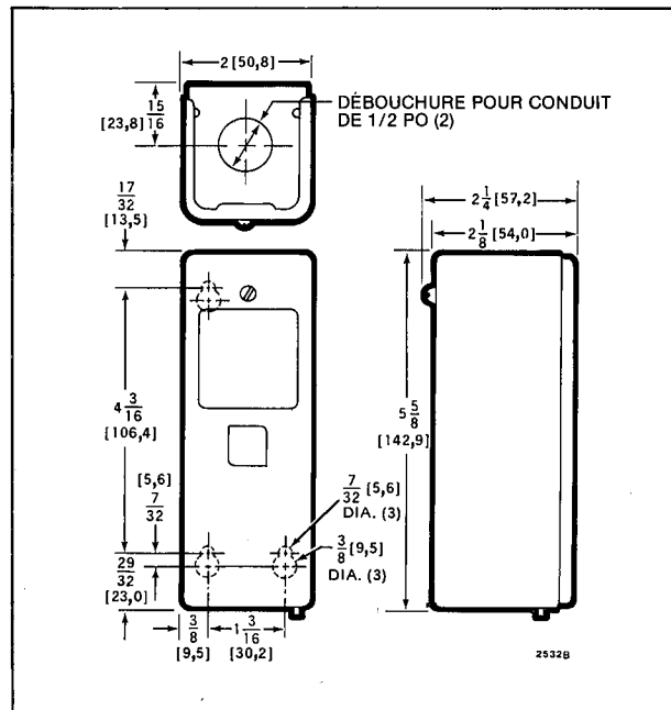
FIG. 1 — DIMENSIONS DES T4031 ET T6031 EN POUCES [mm].
