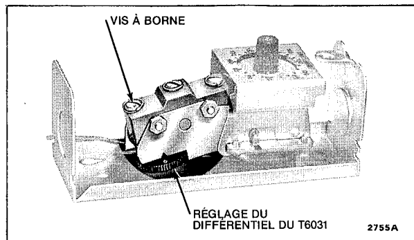
FIG. 7 — VUE INTÉRIEURE MONTRANT LA MOLETTE DE RÉGLAGE DU DIFFÉRENTIEL (POUR CERTAINS MODÈLES).
