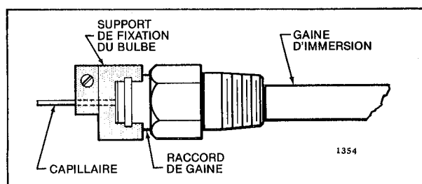
FIG. 4 — GAINE D'IMMERSION.
