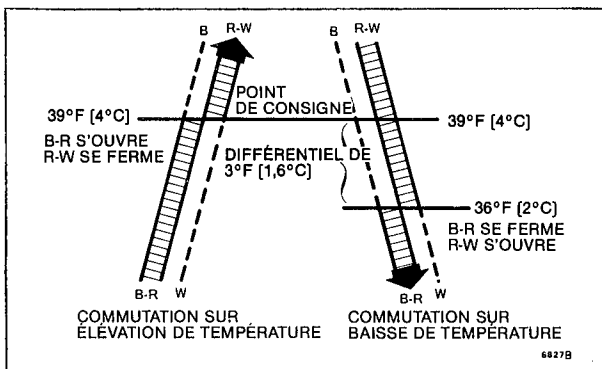
FIG. 6 — COMMUTATION SUR ÉLÉVATION ET BAISSÉ DE TEMPÉRATURE.
