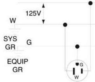
5-15P
