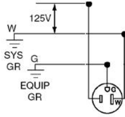
5-15R
