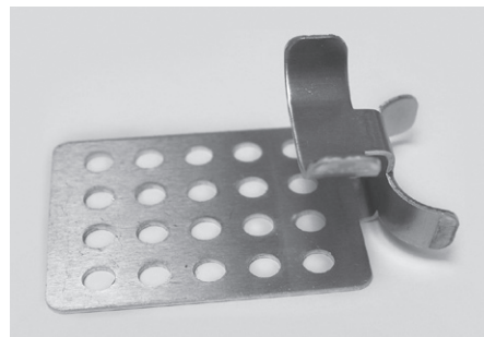
ELB-RCLIP : Attaches de fixation pour toiture, pour maintenir le câble en place sur la toiture. Vis et revêtement étanche non inclus.
